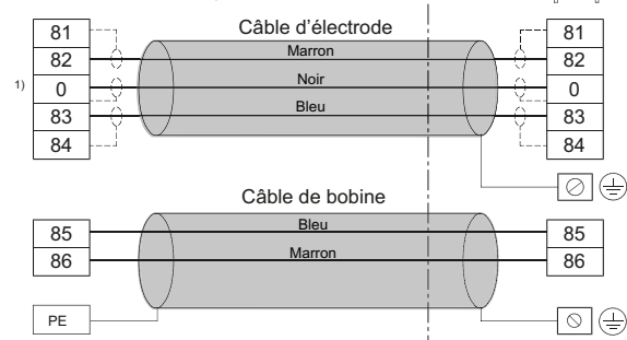
Figure 5-1 Schéma de câblage
